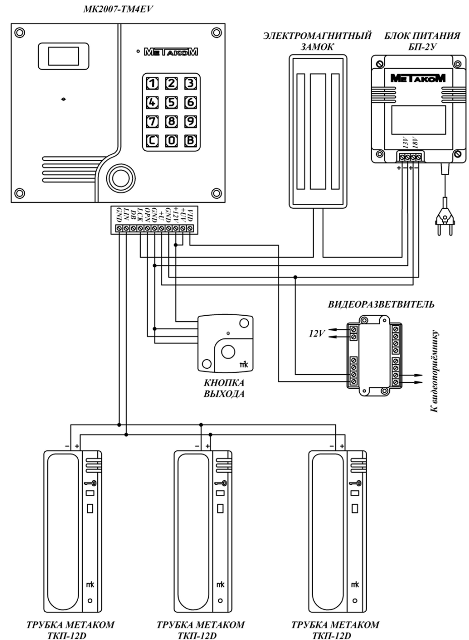
Рис. 2 Пример монтажа блока вызова МК2007-ТМ4ЕV
