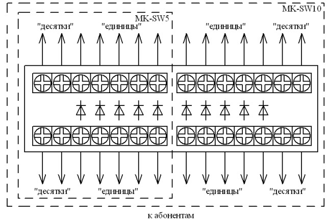
Рисунок 1. Схема подключения разветвителя трубок METAKOM MK-SW10 (МК-SW5).
