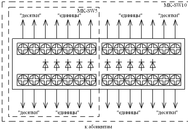
Рисунок 1. Схема подключения разветвителя трубок METAKOM MK-SW10 (МК-SW5).
